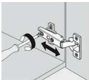
Rys. 3. Regulacja głębokości frontu.
