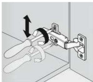
Rys. 1. Regulacja wysokości frontu.
