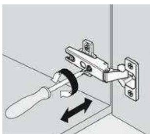
Rys. 2. Regulacja boczna frontu.
